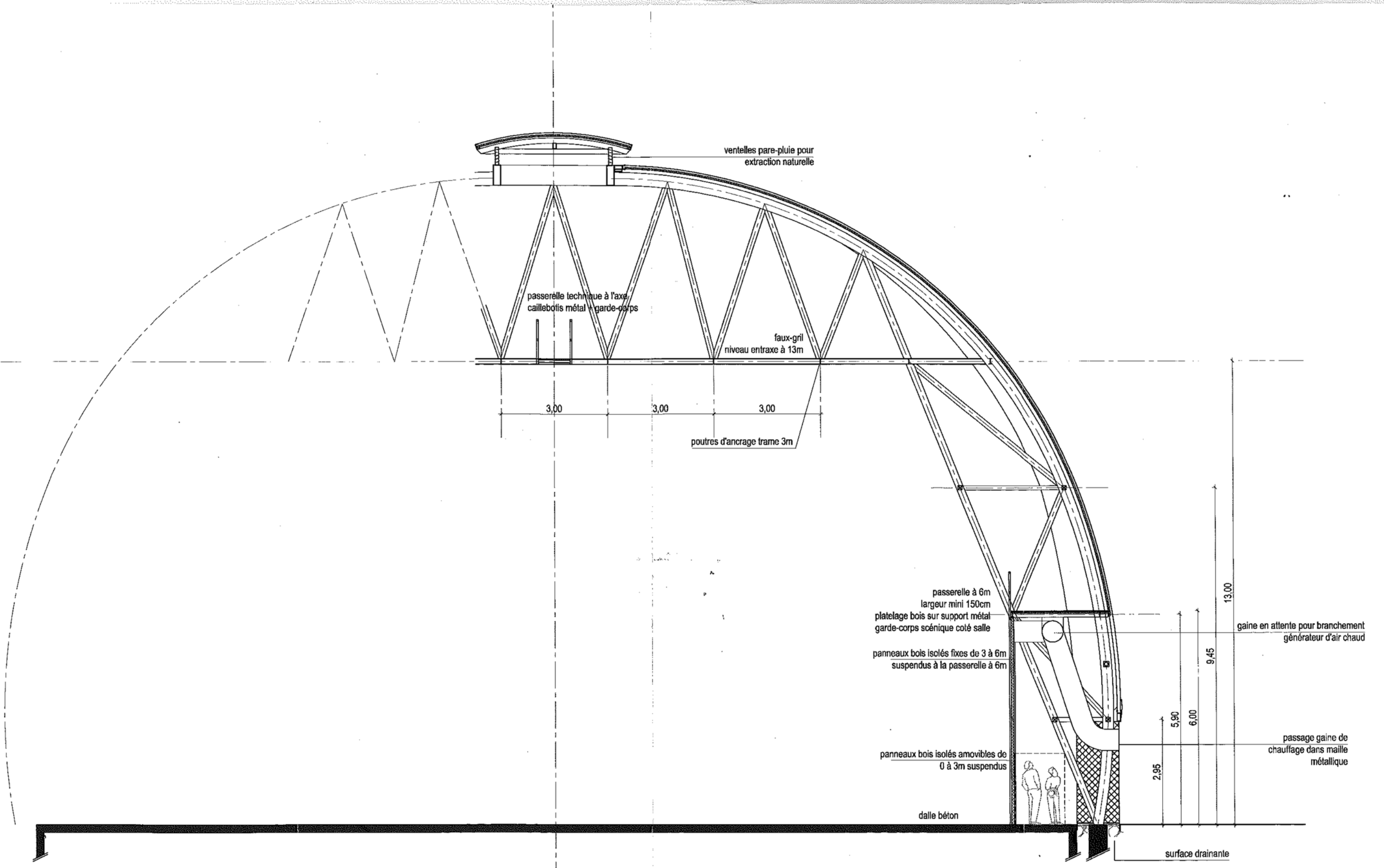
COUPE TRANSVERSALE
